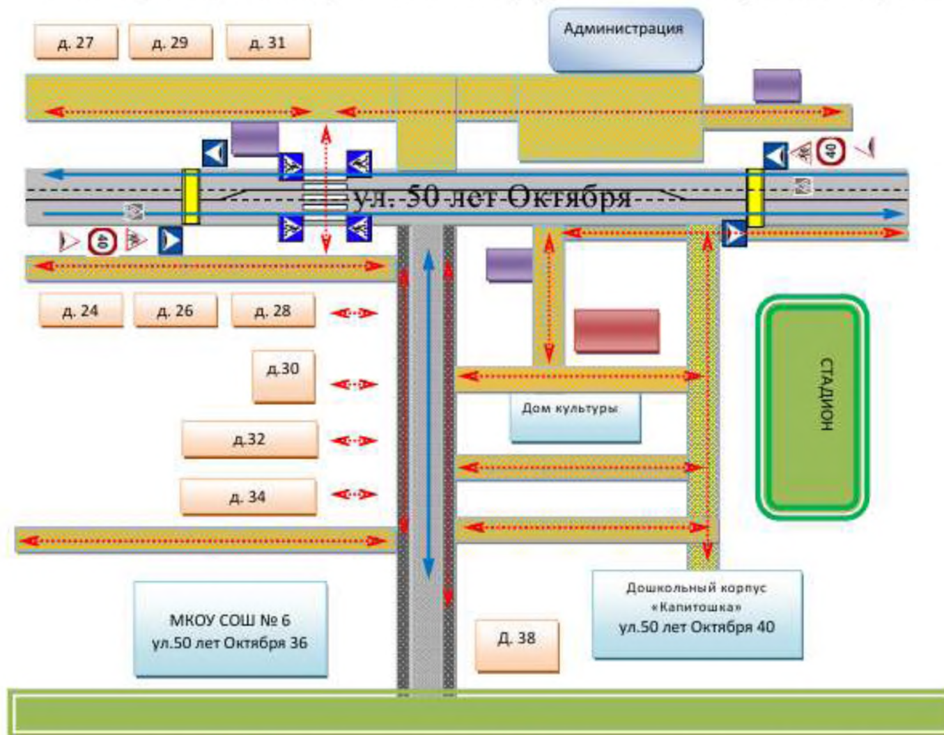
2.Схема организация дорожного движения в непосредственной близости от дошкольного корпуса «Капитошка» с размещением соответствующих технических средств организации дорожного движения, маршрутов движения детей и расположение парковочных мест.
